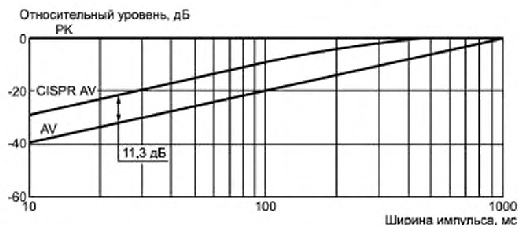
Рисунок С.4 — Пример весовых функций (импульс 1 Гц) при детектировании пиковым детектором «РК» и детектором средних значений «AV» относительно ширины импульсов для постоянной времени прибора 100 мс
