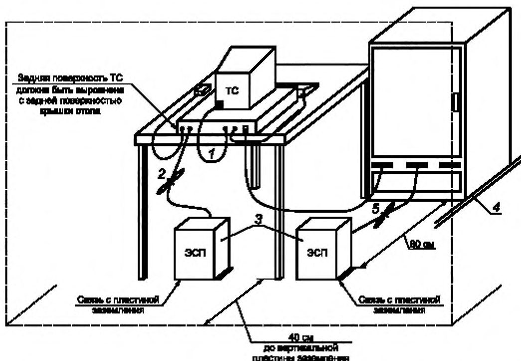
1 — соединительные кабели, удаленные от пластины заземления менее 40 см, уложены в плоские петли (от 30 до 40 см) и вывешены приблизительно в середине между столотом и пластиной заземления, 2 — излишек шнур питания должен быть уложен в связку в виде плоских петель или укорочен до соответствующей длины; 3 — испытуемое ТС подключено к одному ЭСП. ЭСП подсоединяют к вертикальной пластине опорного заземления. На остальное оборудование питание подается от второго ЭСП; 4 — испытуемое ТС и кабели должны быть расположены не ближе, чем 12 мм от горизонтальной пластины опорного заземления, 5 — входной/выходной кабели к наполному блоку опускают по направлению к горизонтальной пластине опорного заземления, а излишек кабелей связывают в виде плоских петель. Кабели, не входящие до горизонтальной пластины опорного заземления, опускают до высоты соединителя или на 40 см, в зависимости от того, что ниже
