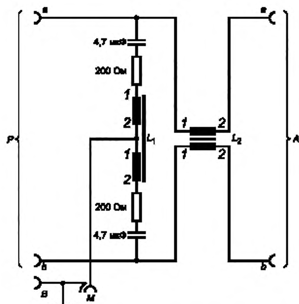
1 — начало обмотки; 2 — конец обмотки; А — зажимы для подключения линии связи; В — зажим опорного заземления; М — вход измерительного приемника (50 Ом); Р — подключение к испытываемому ТС; L_1 — индуктивность симметричного режима (от 5 до 40 мГн для каждой обмотки); L_2 — индуктивность развязки
