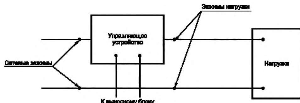
Рисунок 16а — Схема измерения для двухзажимных управляющих устройств
