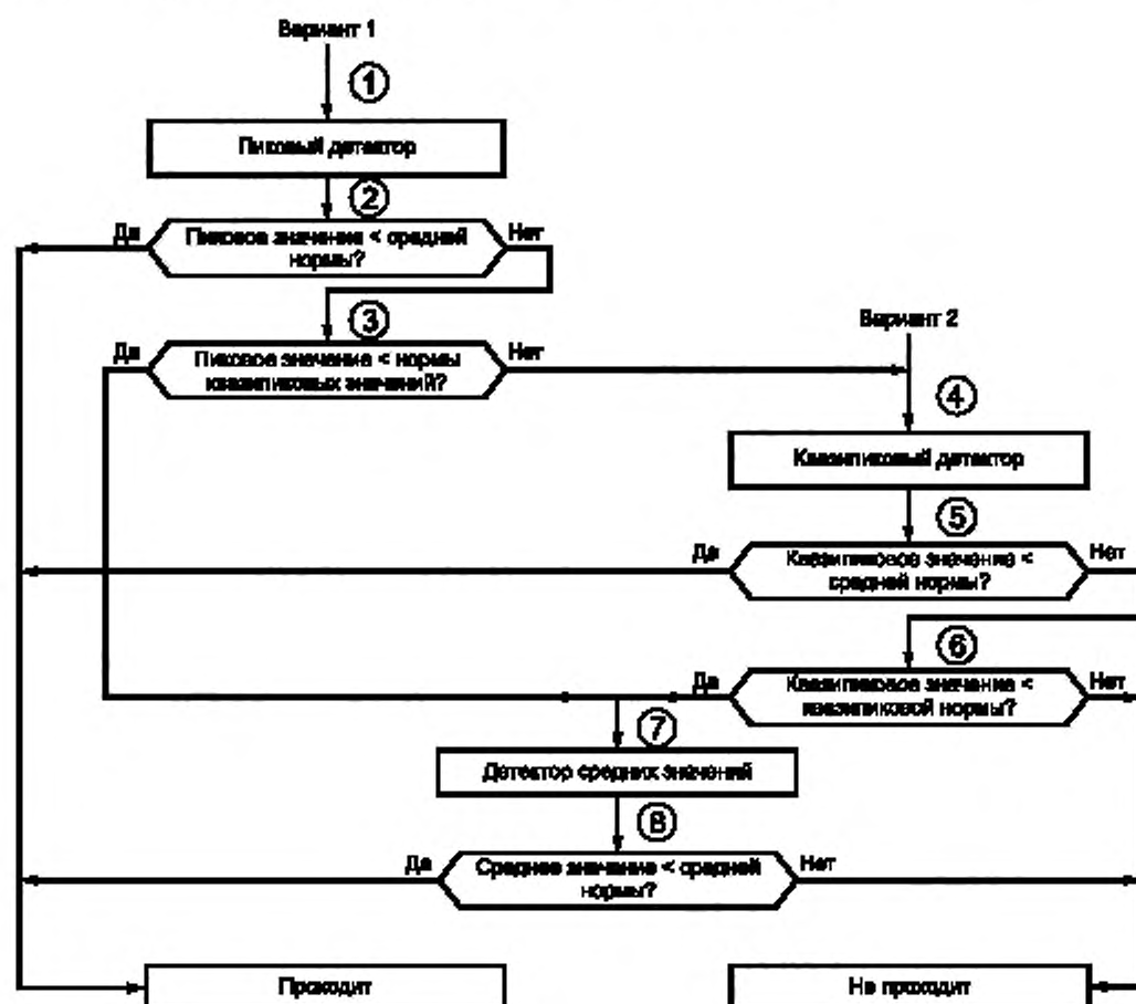
Рисунок С.1 — Алгоритмы определения соответствия ТС нормам кондуктивных ИРП при использовании пикового, квазипикового детектора и детектора средних значений
