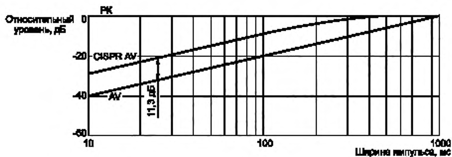
Рисунок D.4 — Пример весовых функций (импульс 1 Гц) при детектировании пиковым детектором РК и детектором средних значений AV относительно ширины импульсов для постоянной времени прибора 100 мс
