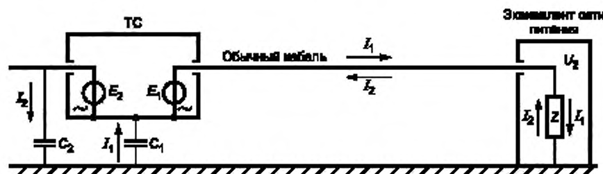
Рисунок А.7 — Поддача питания через неэкранированные провода (эквивалентная схема 7)
