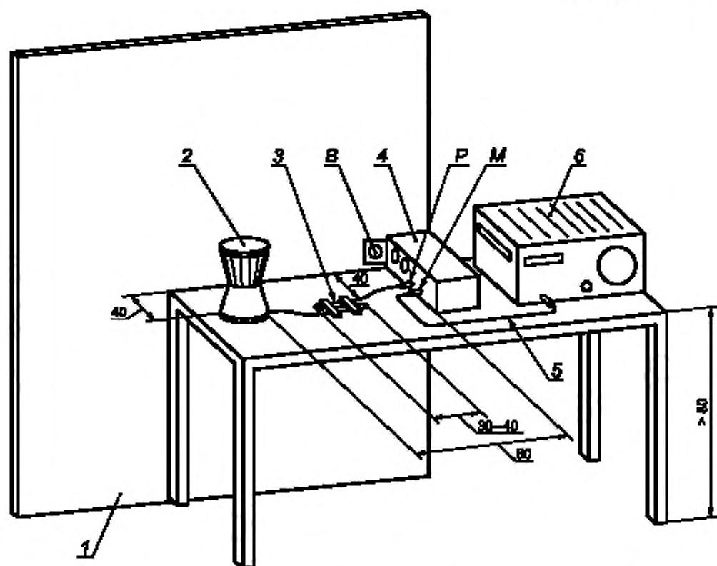
1 — металлическая стена 2 × 2 м; 2 — испытуемое ТС; 3 — излишек сетевого шнура, уложенный плоскими петлями 3 × 40 см; 4 — V-образный эквивалент сети; 5 — коаксиальный кабель; 6 — измерительный приемник; B — соединение с опорным заземлением; M — вход измерительного приемника; P — питание испытуемого ТС
