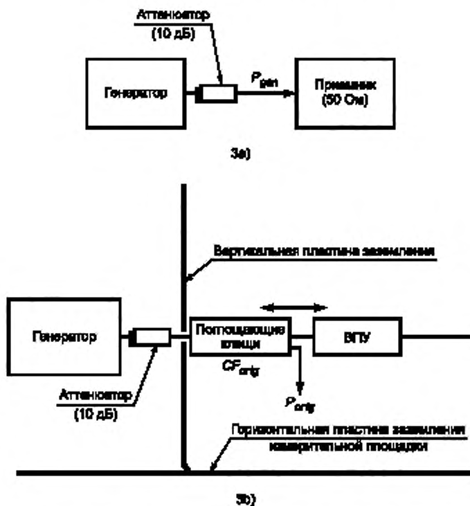
Рисунок 3, лист 1 — Структурные схемы методов калибровки
