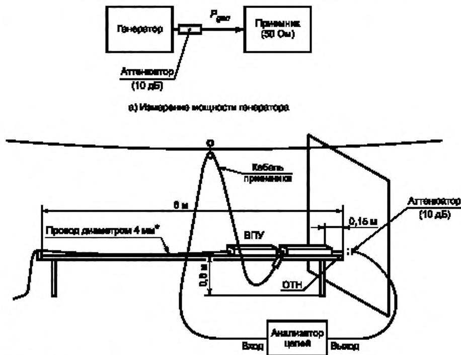
б) Установка для измерения мощности на выходе поглощающих клещей
