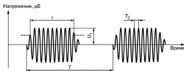
\tau — ширина импульса (на уровне 50 % U_1 ); f_p = 1/T — частота повторения импульсов; f_0 = 1/T_0 — частота несущей сигнала
