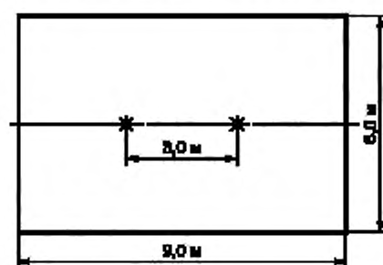
Рисунок 11 — Размеры измерительной площадки
