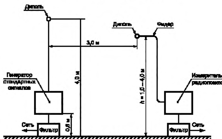
Рисунок 12 — Расположение аппаратуры при измерении площадки
