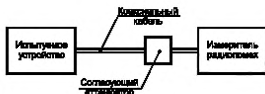
Рисунок 9 — Структурная схема измерения направленности радиопомех и poziomu сигнала на ВЧ-выходе испытуемого устройства
