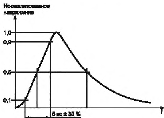
Рисунок 3 — Форма импульсов напряжения на выходе ИГ при нагрузке 50 Ом
