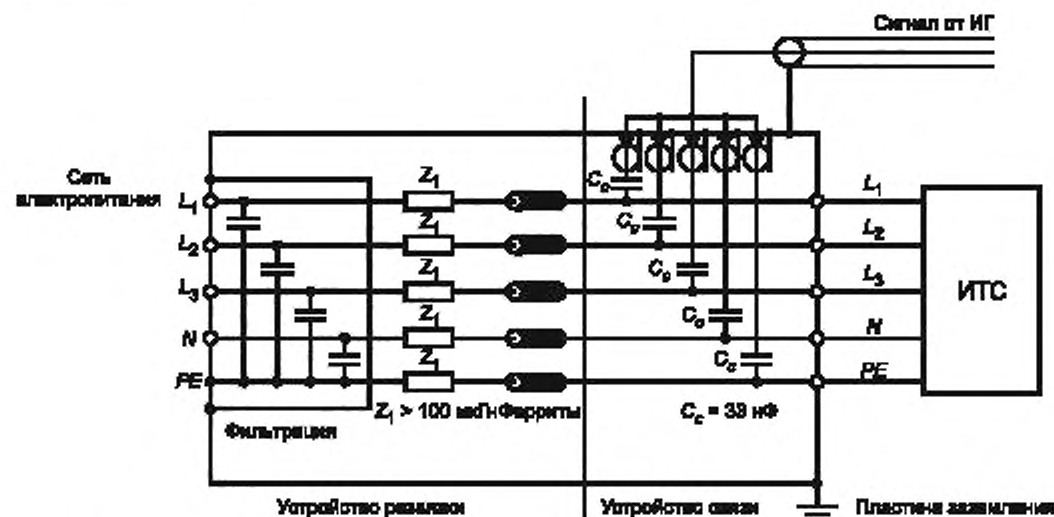
Рисунок 4 — Пример устройства связи/развязки для подачи НИП на порты электропитания переменного и постоянного тока
