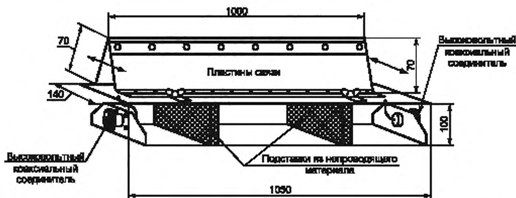
Рисунок 5 — Конструкция емкостных клещей связи
