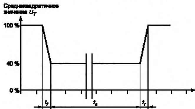
t_r — время нарастания напряжения, t_p — время понижения напряжения; t_s — время выдержки на пониженном напряжении
