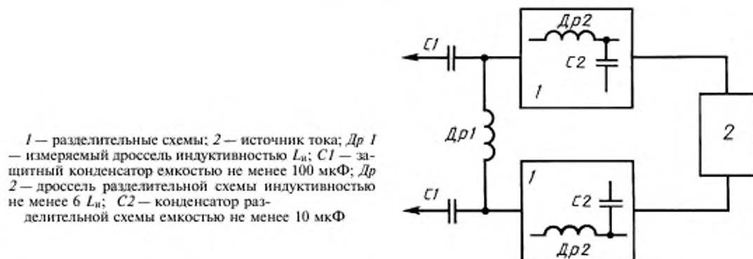
Измерительная схема
