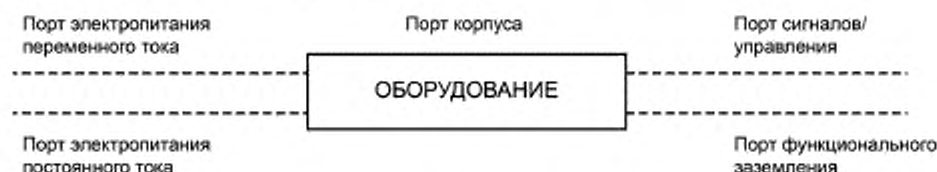
Рисунок 1 — Примеры портов
