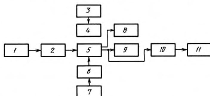
Структурная схема измерений уровня помехозащищенности приемника по отношению к электромагнитному полю
