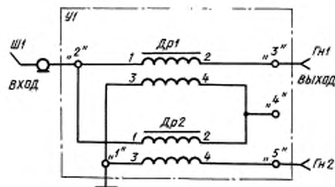
Схема электрическая принципиальная согласующего устройства Е-установки
