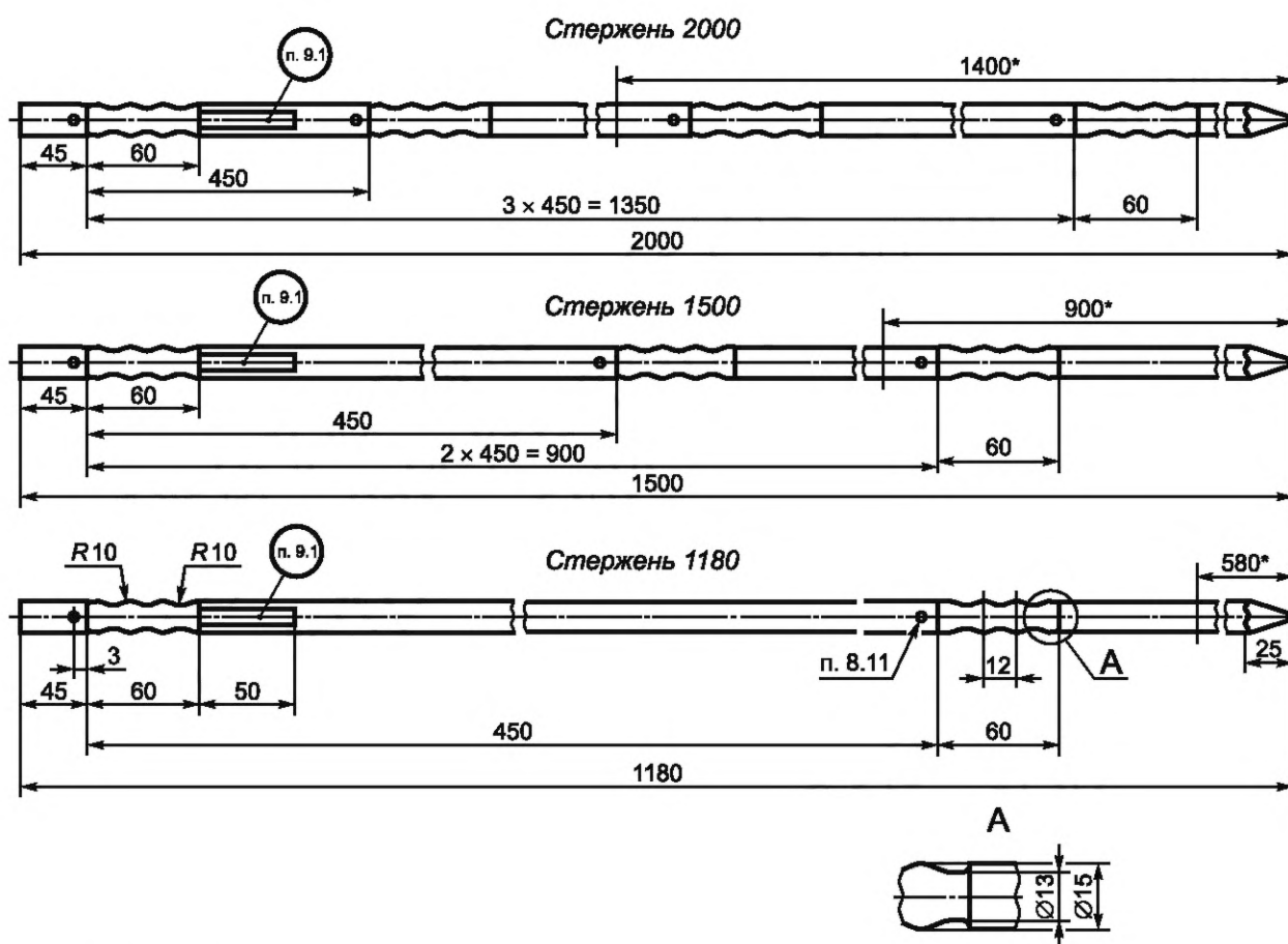
Рисунок 2 — Стержни
