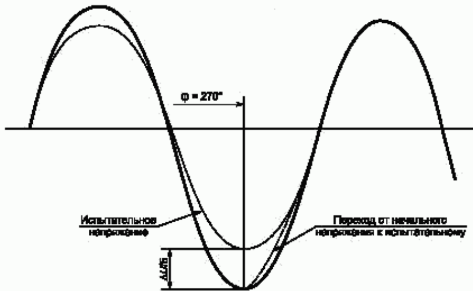
Рисунок 1в — Изменение напряжения в течение 0,25 периода при образовании t_r и t_d
