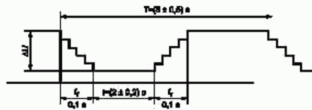
Рисунок 1б — Определение времени спада t_d и времени возрастания t_r при формировании ступенчатых изменений напряжения
